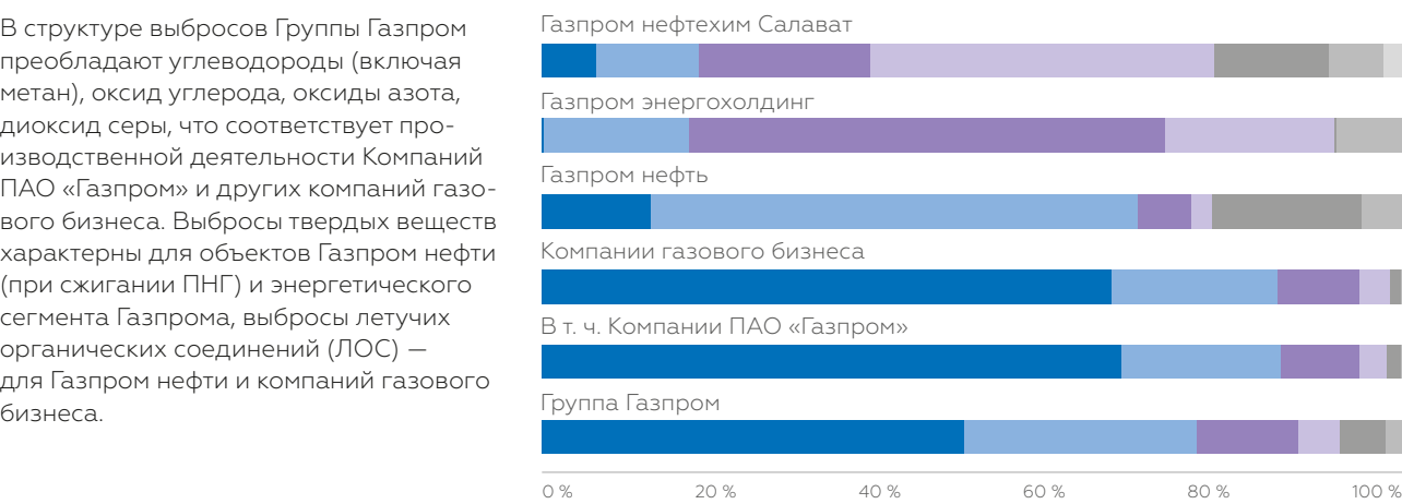
Компонентная структура выбросов в атмосферный воздух в Группе Газпром, 2024 г., тыс. т, %
