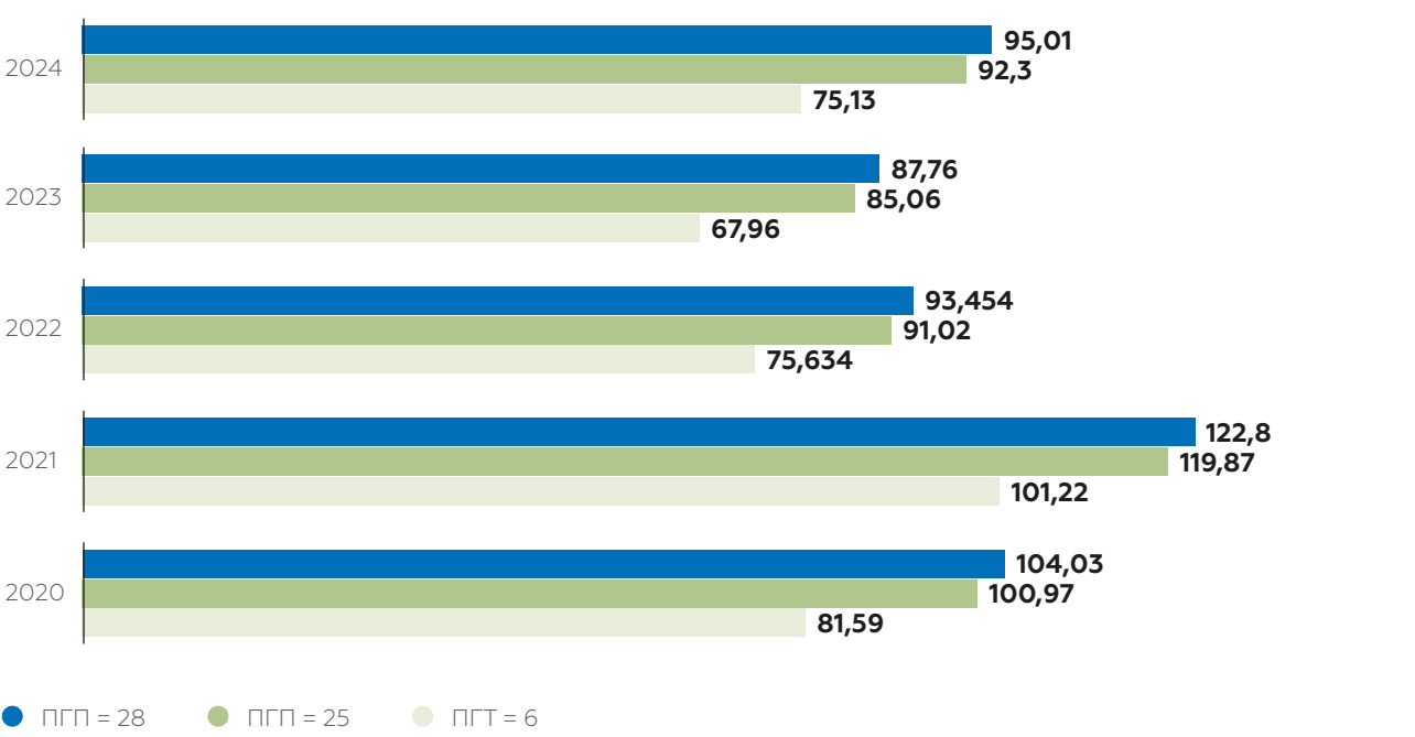
Динамика выбросов ПГ Компаний ПАО «Газпром», 2020–2024 гг., млн т CO 2 -экв.
