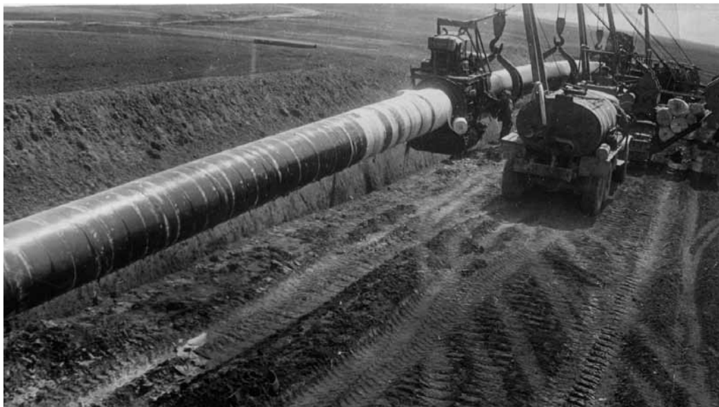
Строительство газопровода в Саратовской области ведется по заказу СДСГ
